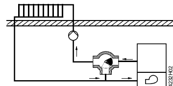
Départ chaudière à droite
