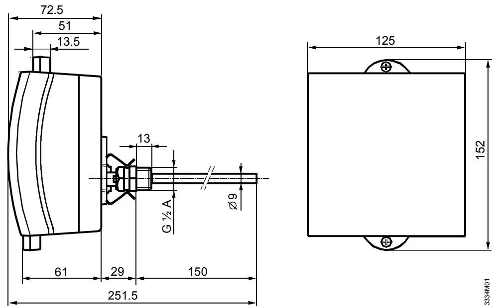
Régulateur avec gaine de protection
